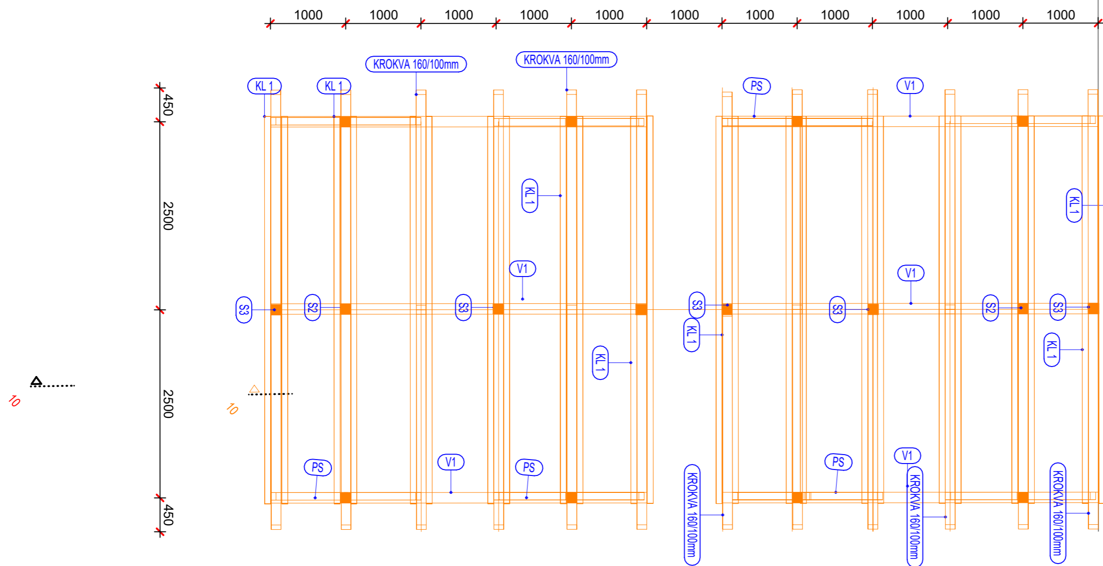
VÝKAZ KROVU ALTÁNOV č.1 Ač2
